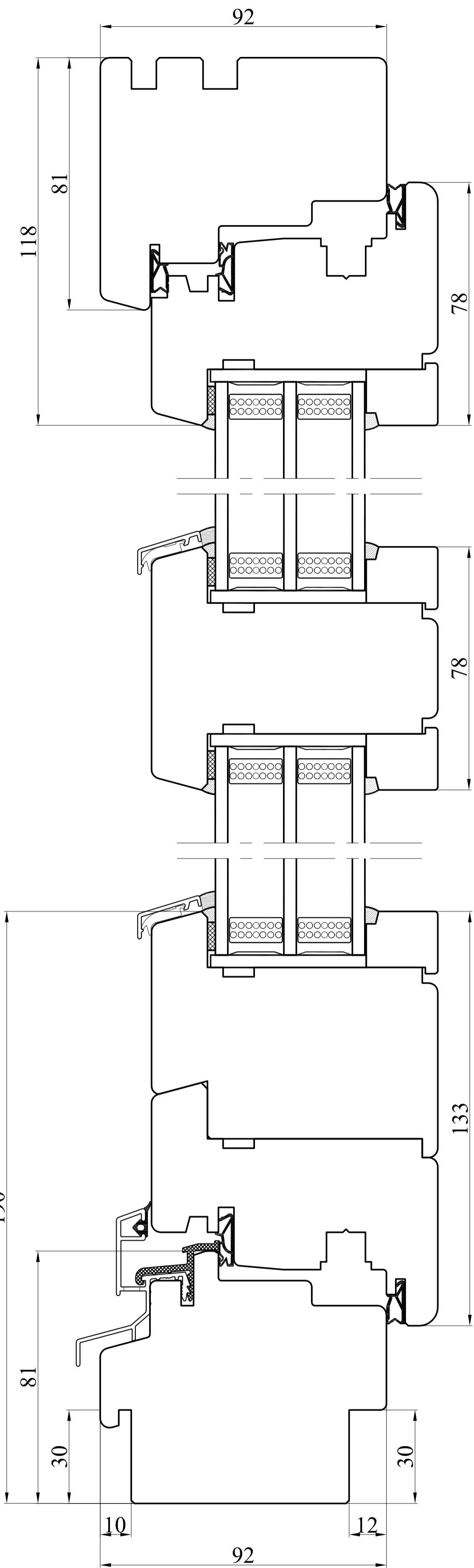
Przekrój A-A
