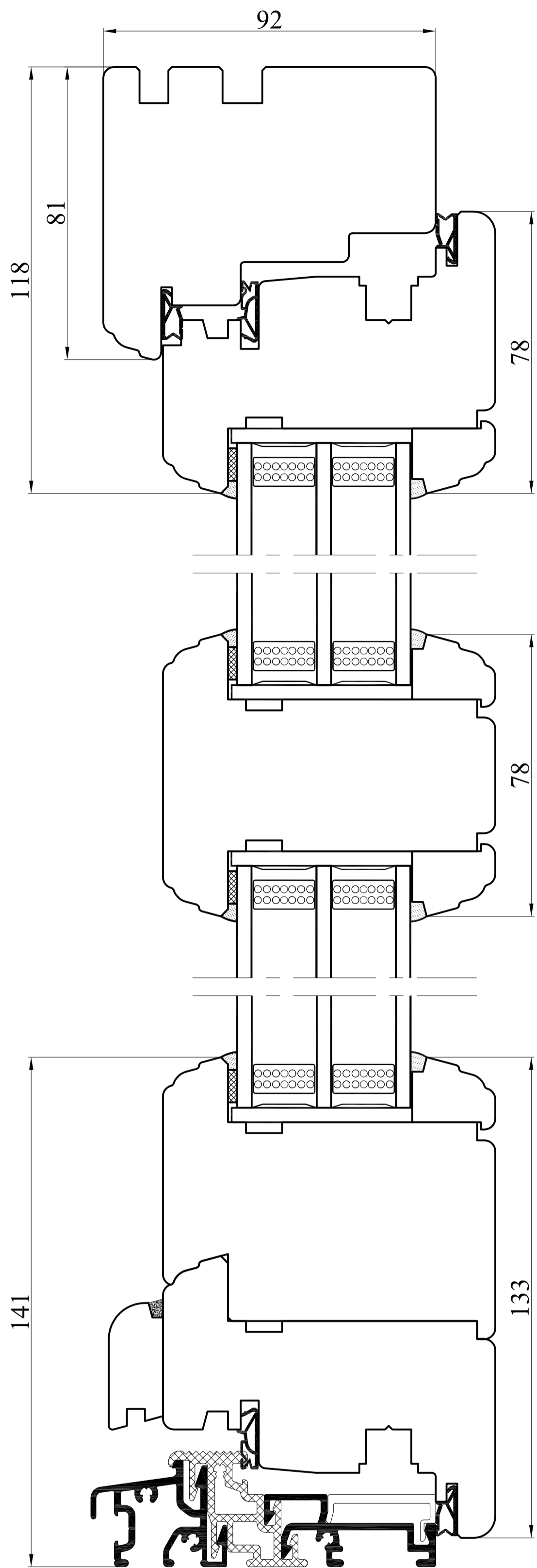
Przekrój A-A
