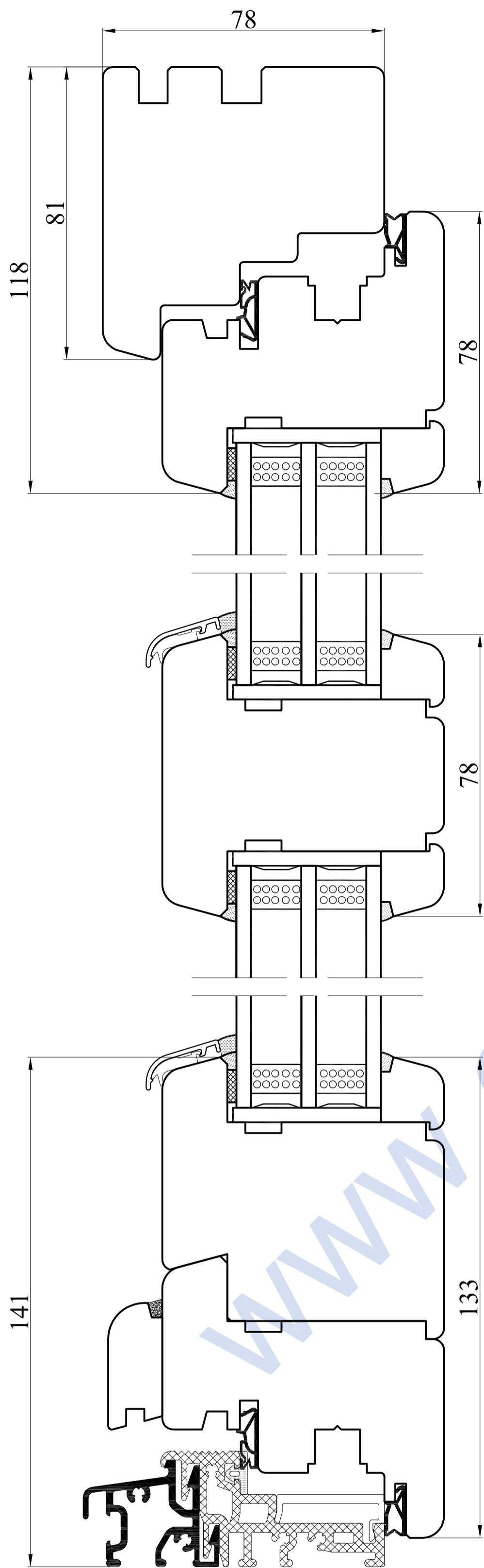
Przekrój A-A
