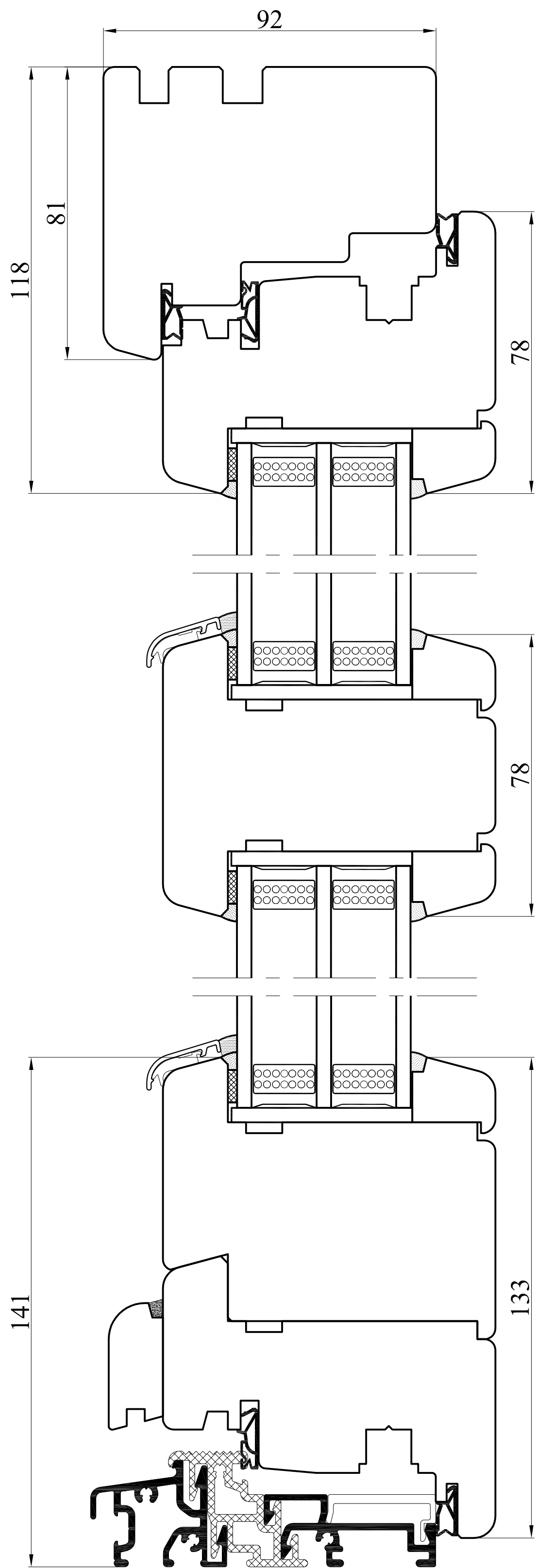
Przekrój A-A
